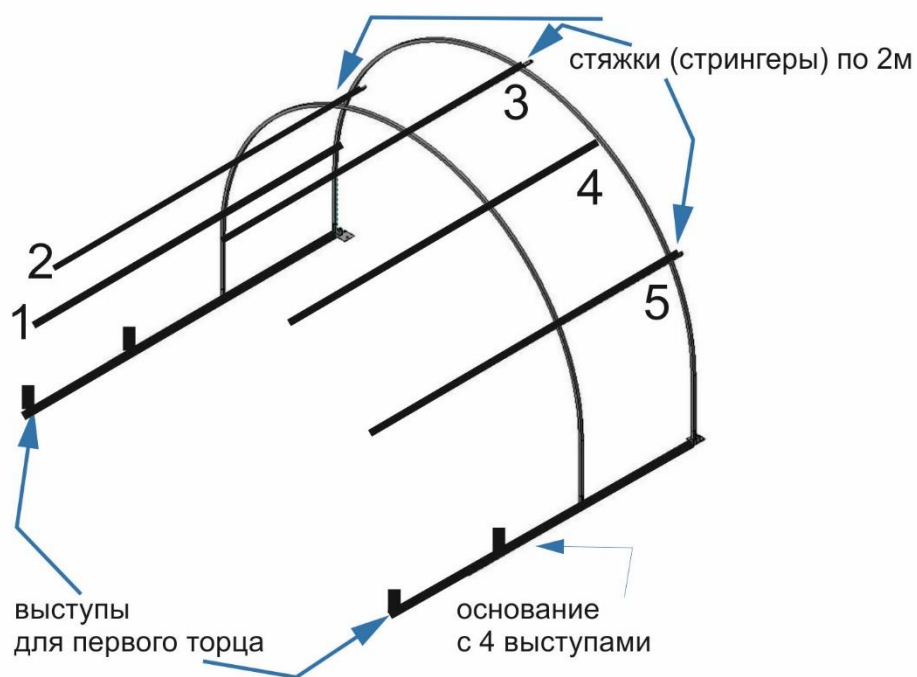
Фото №2. Стяжки (стрингеры) в шахматном порядке.
