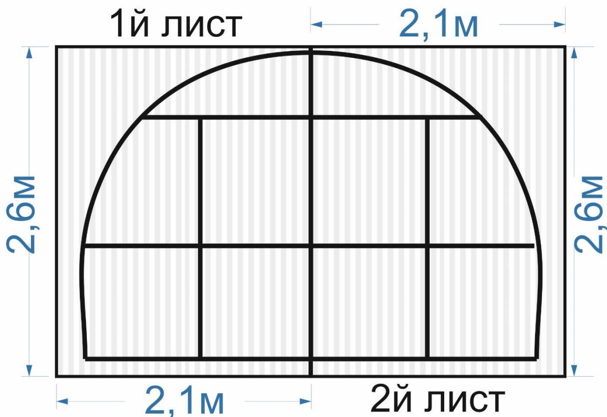
Рисунок №1. Схема раскроя поликарбоната на торцы
